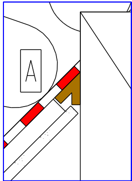
uszczelnienie płatwi taśmą SIGA Corvum 30/30
