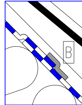
zakłady membrany paroprzepuszczalnej uszczelnione taśmą SIGA Wigluv
